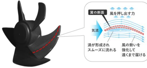
フクロウの翼形状を応用し 断面にふくらみを持たせたファン
